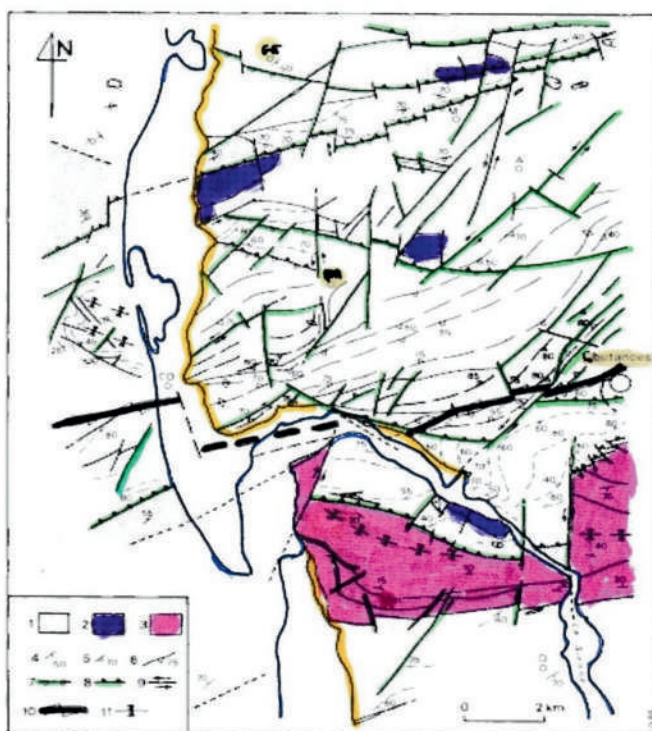
Fig. 7 - Schéma structural de la feuille Coutances
